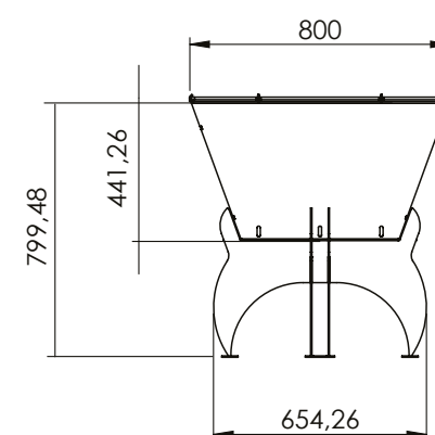
PESO GRINGO con base Spider Gewicht Gringo mit Unterbau Spider 110 kg
