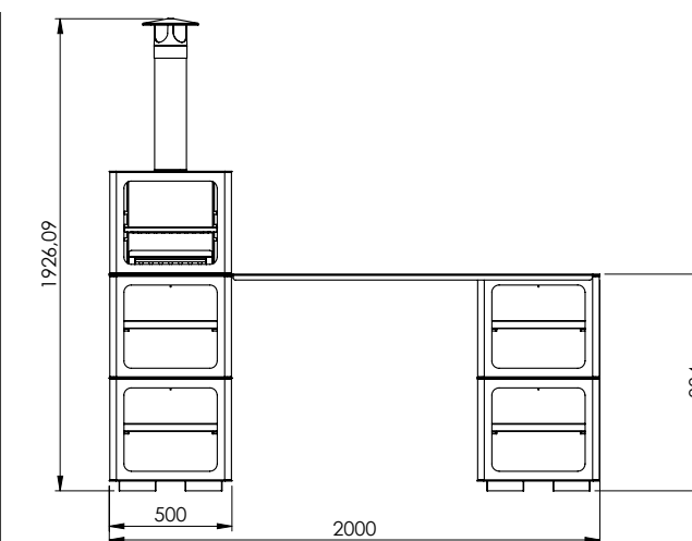
TOTEM PLUS - 180 kg
