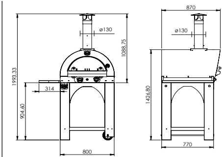
PULCINELLA GAS 60x60 cm - 150 kg 1 bruciatore di serie Serienausstattung 1 Brenner
