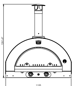
FAMILY GAS 100x80 cm - 240 kg 2 bruciatori di serie Serienausstattung 2 Brenner
