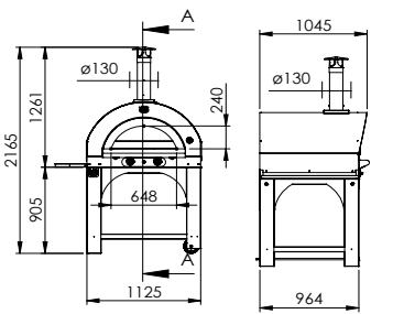
PULCINELLA GAS 100x80 cm - 295 kg 2 bruciatori di serie Serienausstattung 2 Brenner
