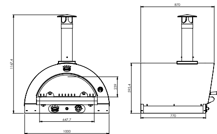
FAMILY GAS 80x60 cm - 135 kg 1 bruciatore di serie + optional aggiuntivo Serienausstattung 1 Brenner + 1 Zusatzbrenner optional
