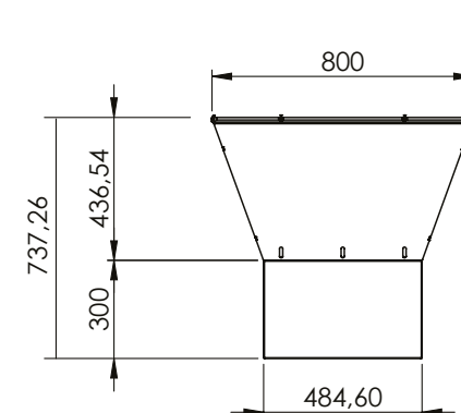
PESO GRINGO con base Cube Gewicht Gringo mit Unterbau Cube 90 kg
