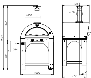
PULCINELLA GAS 80x60 cm - 190 kg 1 bruciatore di serie + 1 optional aggiuntivo Serienausstattung 1 Brenner + 1 Zusatzbrenner optional
