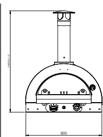
FAMILY GAS 60x60 cm - 115 kg 1 bruciatore di serie Serienausstattung 1 Brenner
